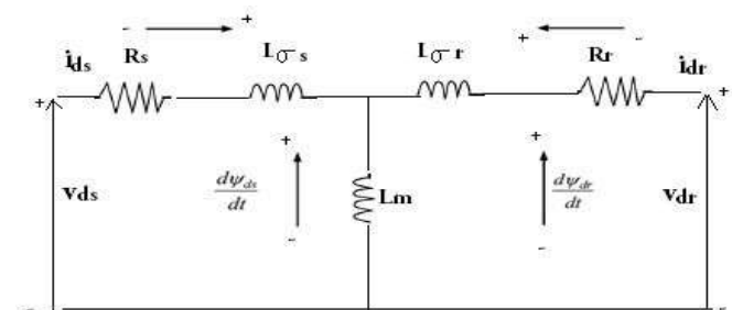
Fig.3.Dynamic d-q axis circuit.
