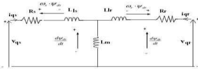
Fig.4. Dynamic q axis circuit.
